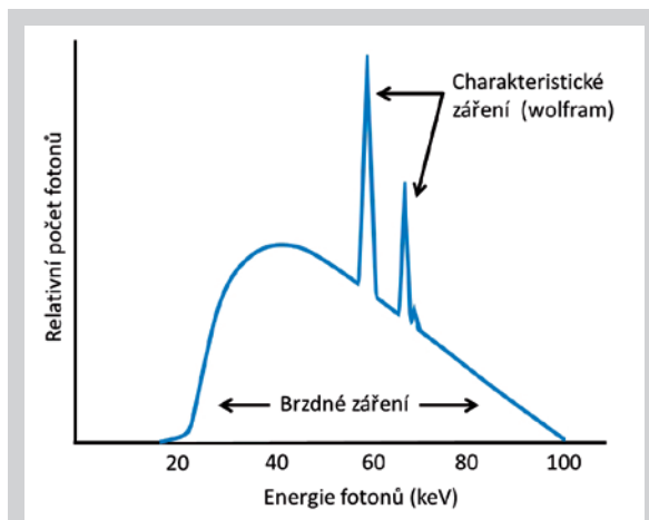
Spektrum rentgenového záření
