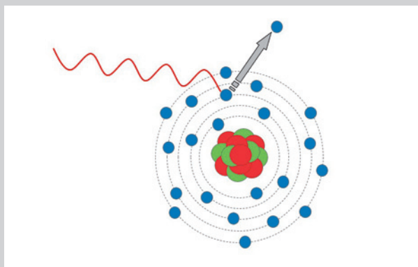
Fotoefekt
